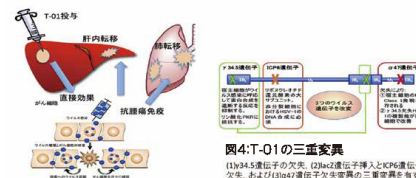
図3: T-01の抗腫瘍効果のメカニズム
